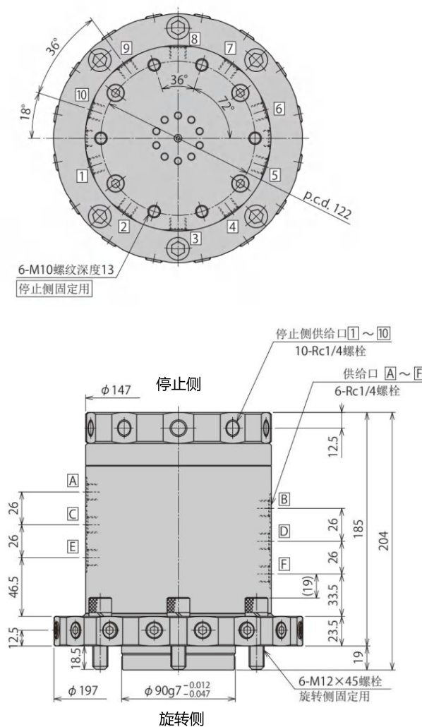
本图表示(16回路)
