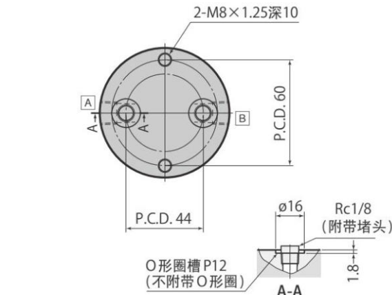
本图表示(2回路)
