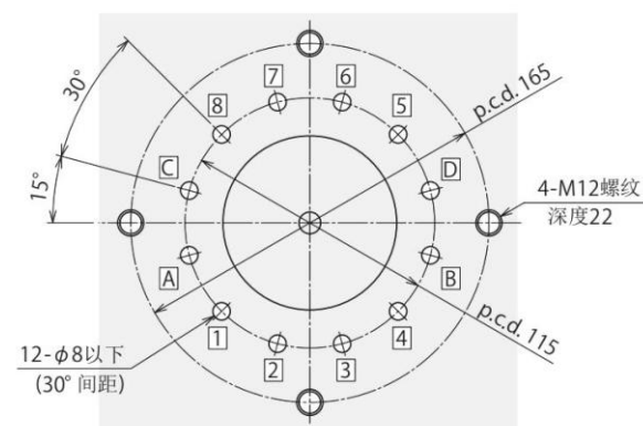
安装部位加工尺寸
