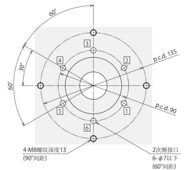
安装部位加工尺寸
