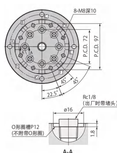
本图表示(8回路)
