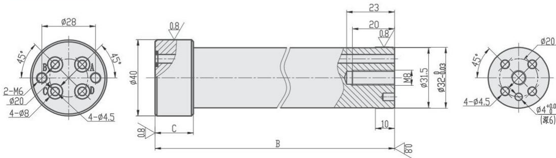
TMG-C-4
