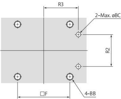
安装孔加工图
