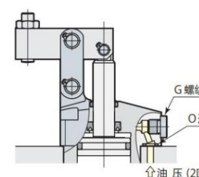
板式连接
