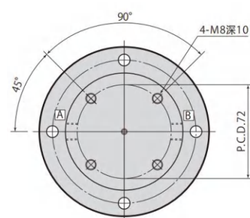
本图表示(2回路)
