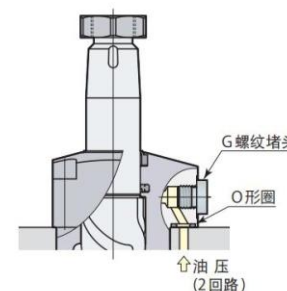
板式连接
