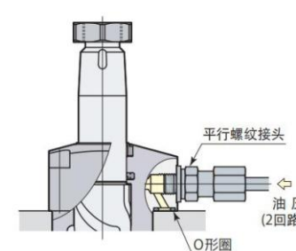
螺纹配管
