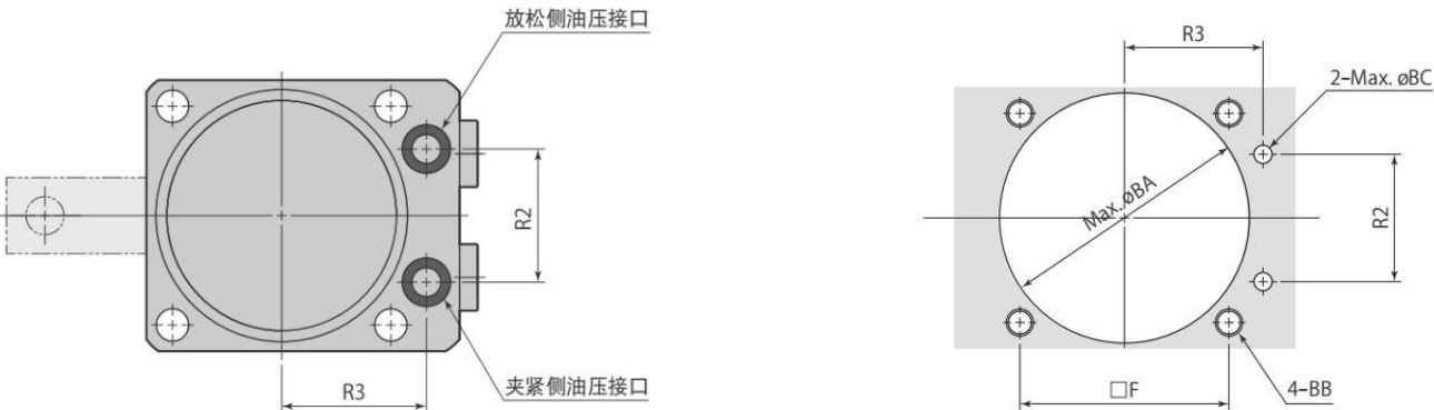
安装孔加工图
