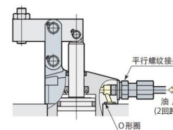
G螺纹配管
