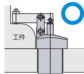
长夹紧臂
