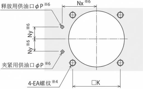
双压臂参考图
