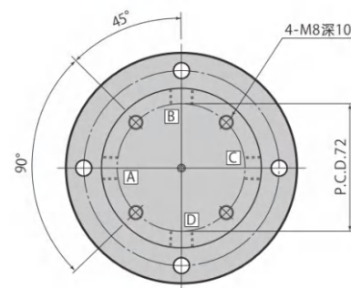
本图表示(4回路)
