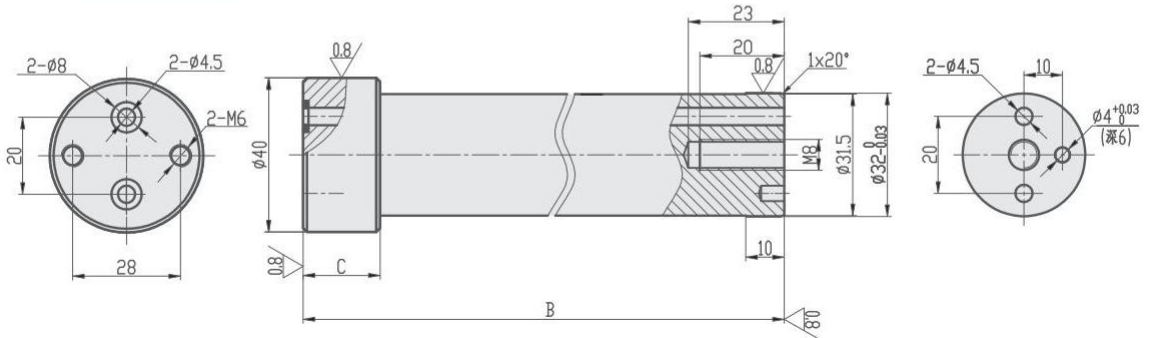
TMG-C-2
