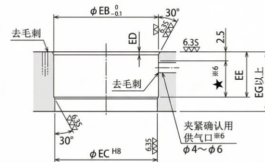
通孔
