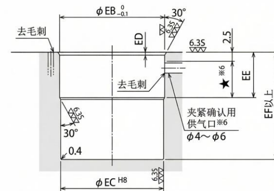
通孔
