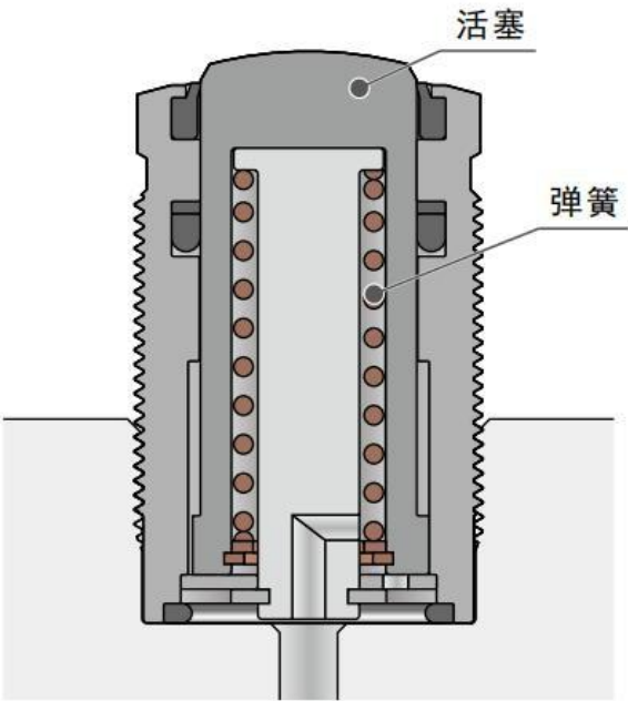
单动型
