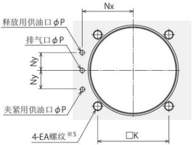
安装孔加工图
