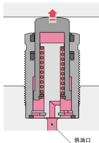
夹紧时
