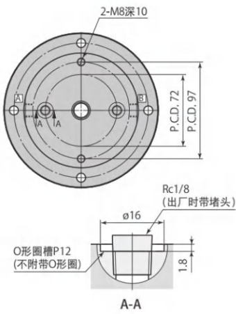
本图表示 (2 回路)
