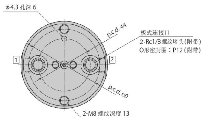
本图表示(2回路)
