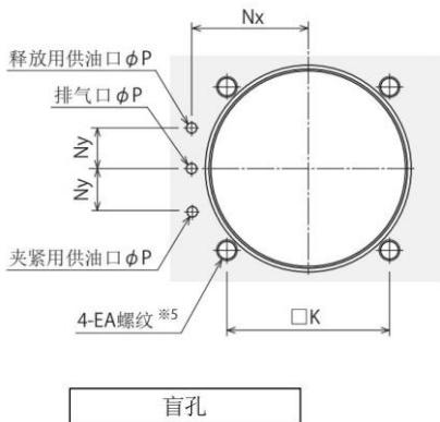
安装部位加工尺寸
