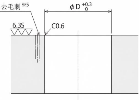
安装孔加工图
