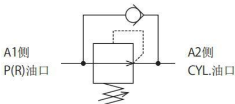
油压无泄漏减压阀 回路符号
