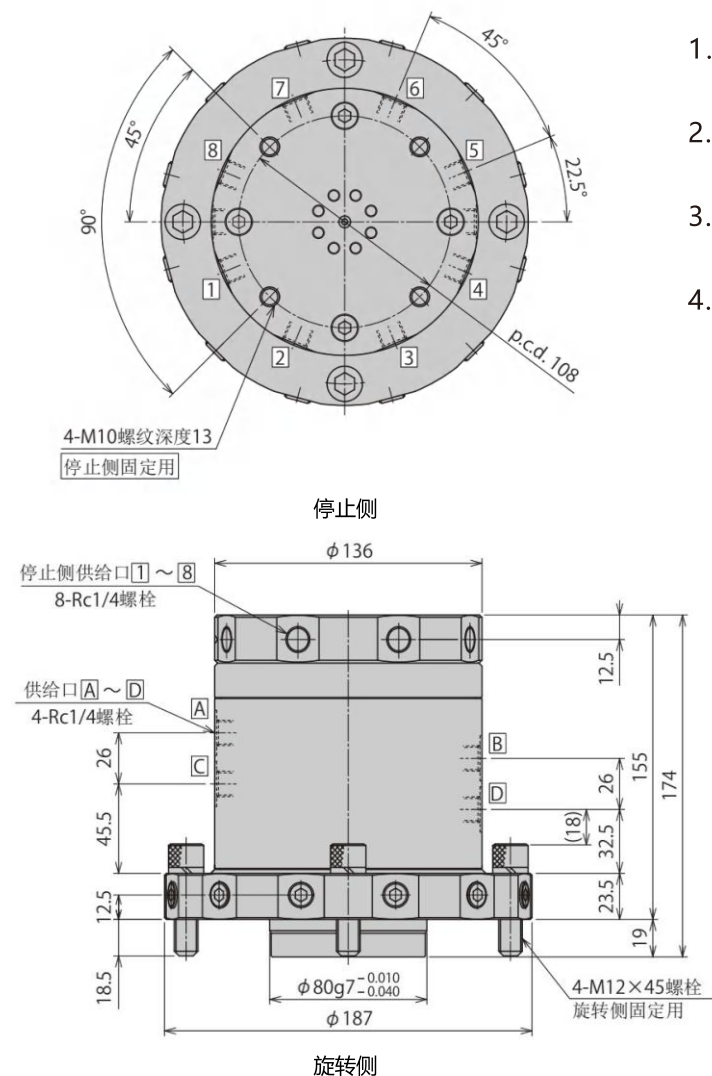
本图表示 (12回路)
