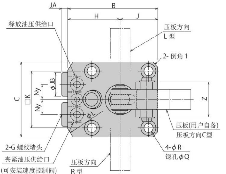
夹紧检测型
