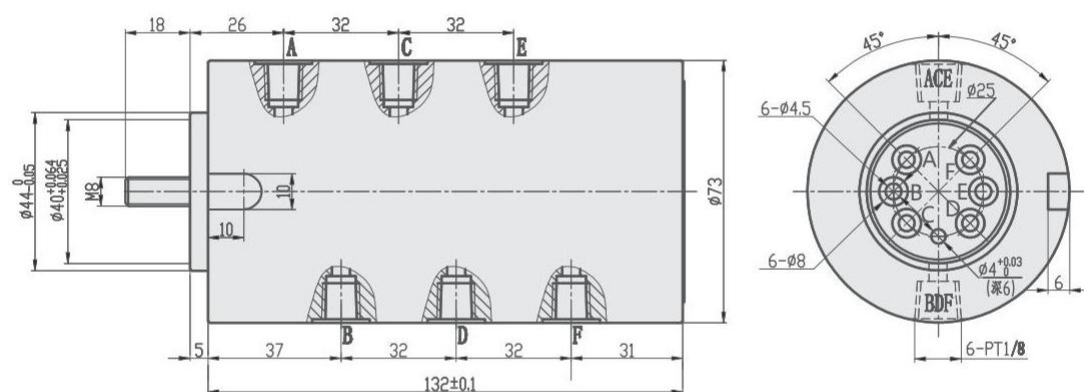
TMG-B-6
