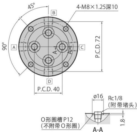
本图表示(4回路)
