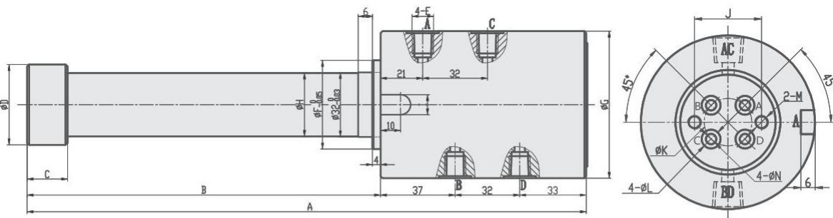
TMG-A-4
