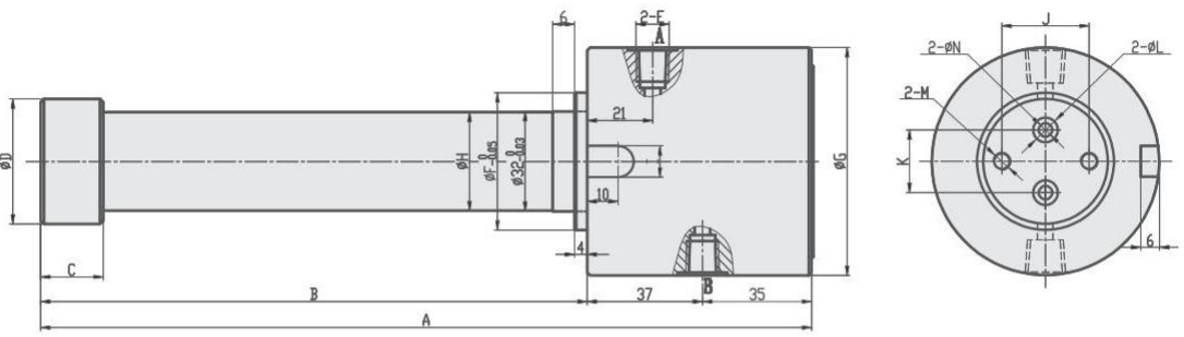
TMG-A-2
