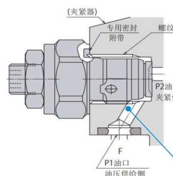
流量控制阀
