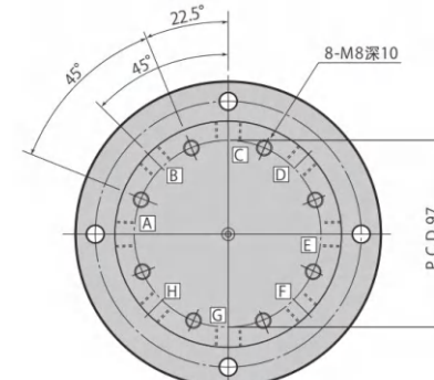
本图表示(8回路)
