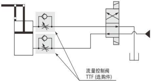
油压回路图
