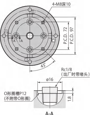
本图表示 (4 回路)
