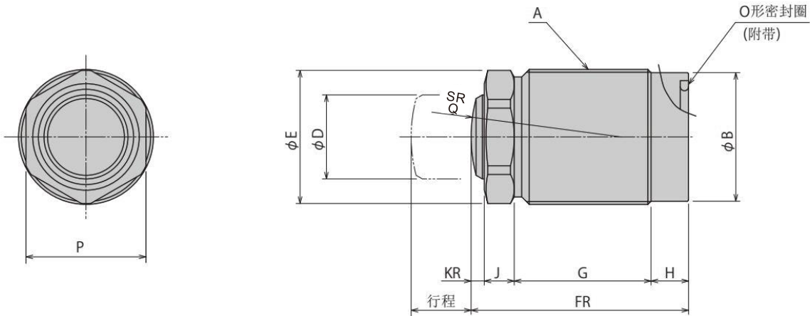
活塞头部形状 R：球面R型
