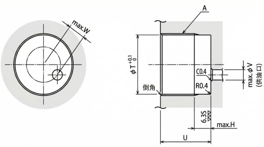
安装部位加工尺寸
