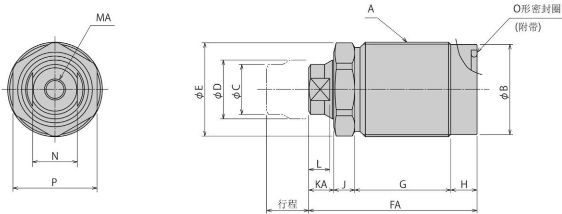
活塞头部形状 A：内螺纹型
