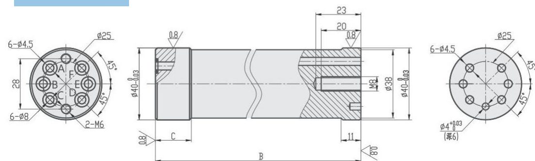
TMG-C-6
