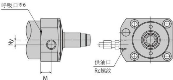
配管方式 S: 外配管型 (Rc 螺纹)
