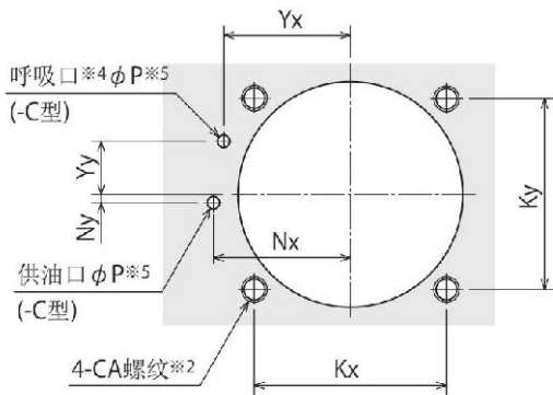
配管方式 S: 外配管型 (Rc 螺纹)
