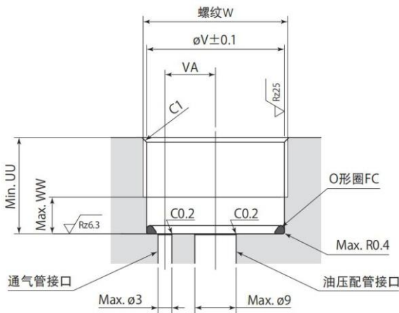
安装孔加工图
