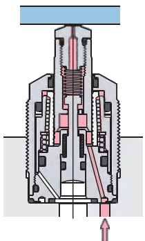
工件接触确认气压
