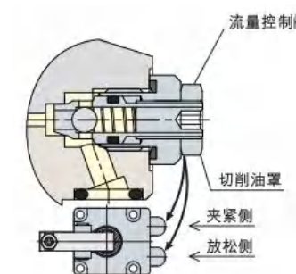
流量控制阀
