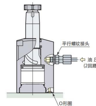
G螺纹配管
