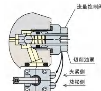
流量控制阀
