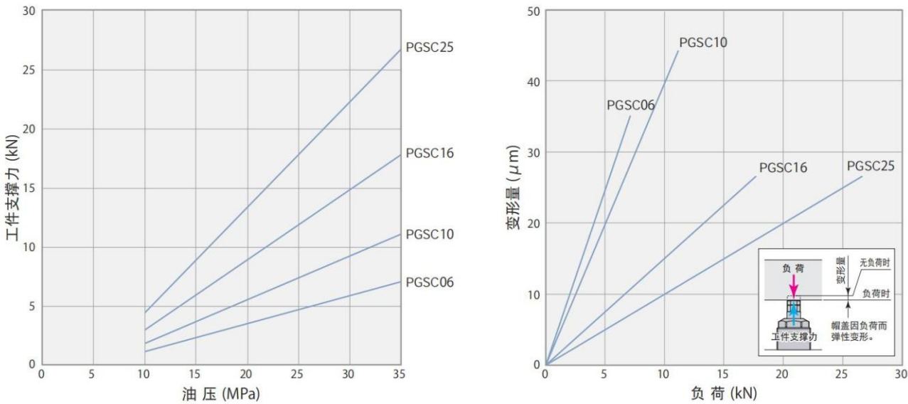
本图表示供给油压35MPa 条件下的静态载荷下的变化
