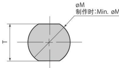
帽盖详图硬度 HRC52
