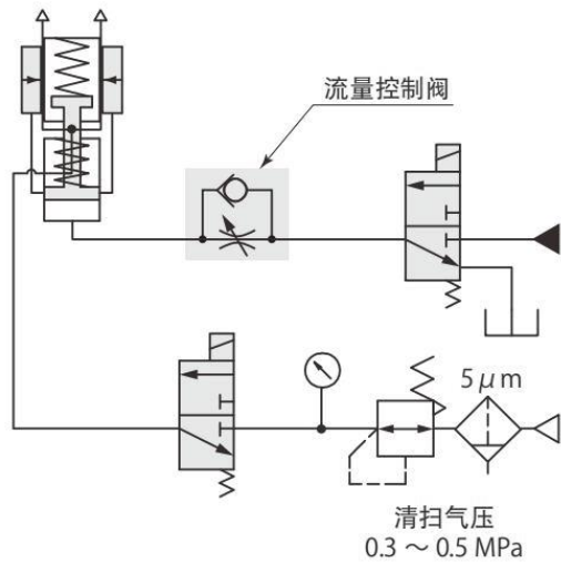
油压、气压回路图
