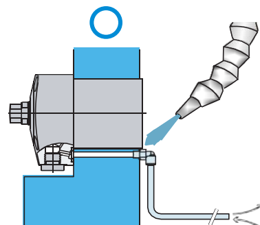
在切削液不影响的地方进行配管
