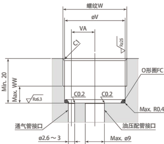
安装孔加工图
