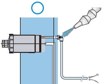
在切削液不影响的地方进行配管
