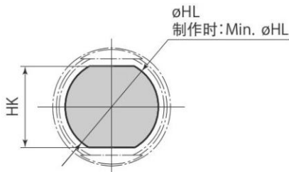
帽盖详图硬度 HRC52
