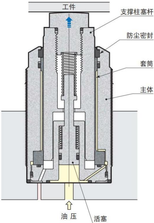
横截面剖析图
