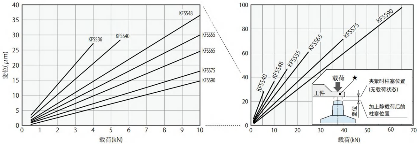
本图表示供给油压 7MPa 条件下的静态载荷下的变化
