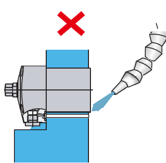
通气孔进入切削液
