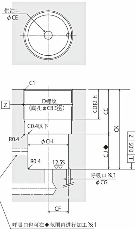
安装孔加工图
