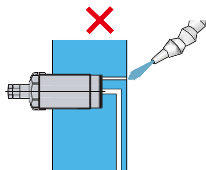
通气孔进入切削液
