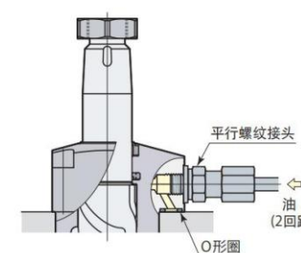
G螺纹配管
