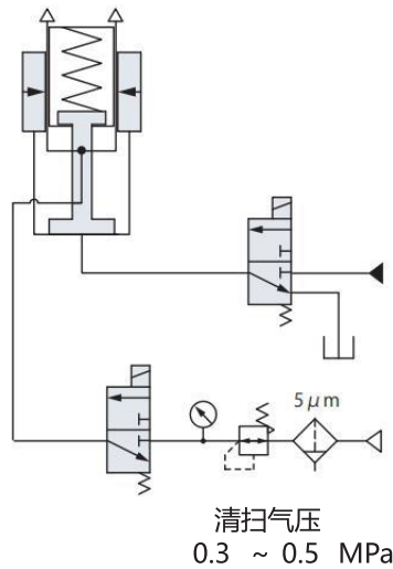
油压、气压回路图
