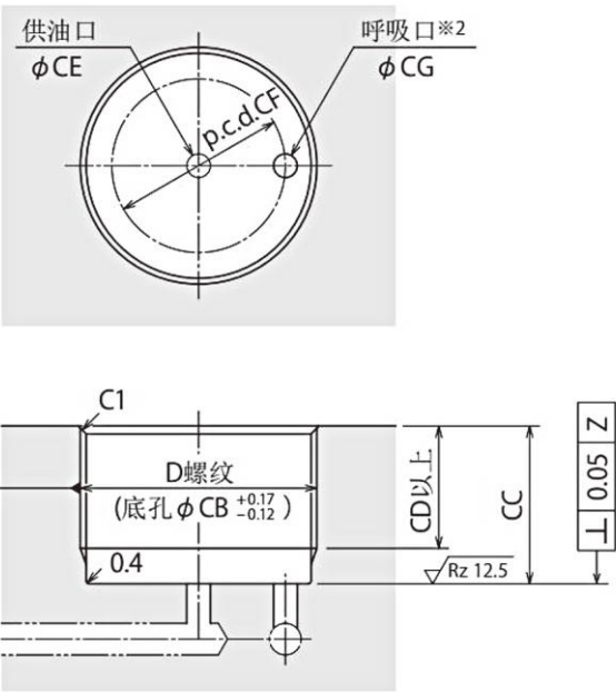
安装孔加工图
