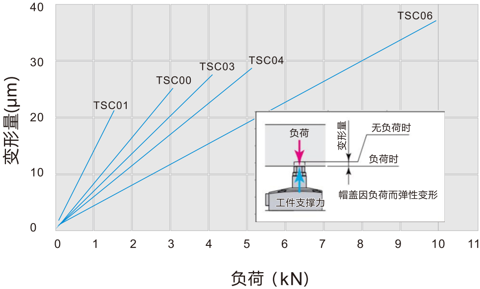
本图表示供给油压7MPa条件下的静态载荷下的变化
