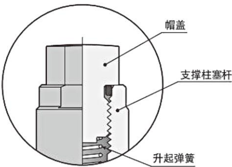
支撑柱塞杆顶端部详图
