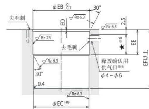
盲孔
