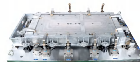
杠杆缸应用
