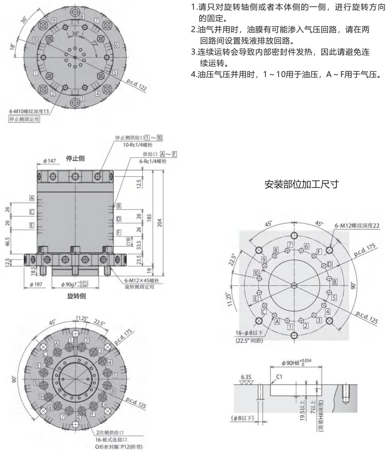
本图表示(16回路)
