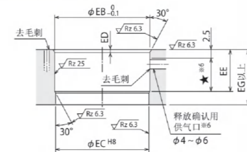
通孔
