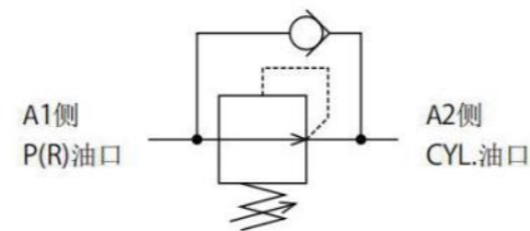
油压无泄漏减压阀 回路符号
