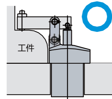
长夹紧臂
