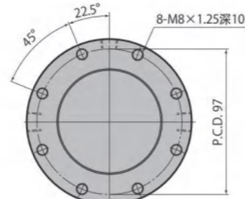
各配管接口处刻有A~H记号
