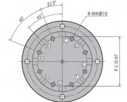
本图表示(8回路)
